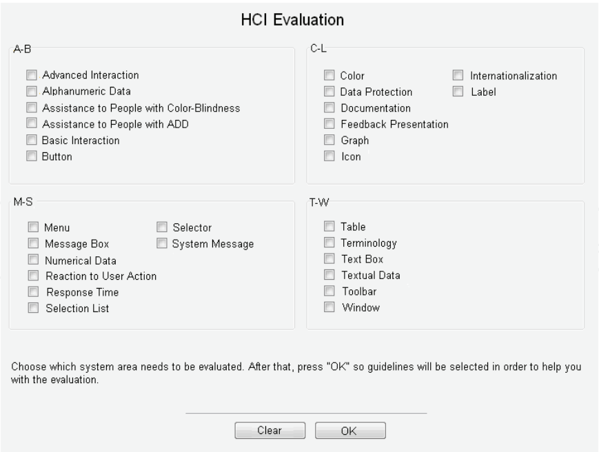
Fig. 6. HCI evaluation.
