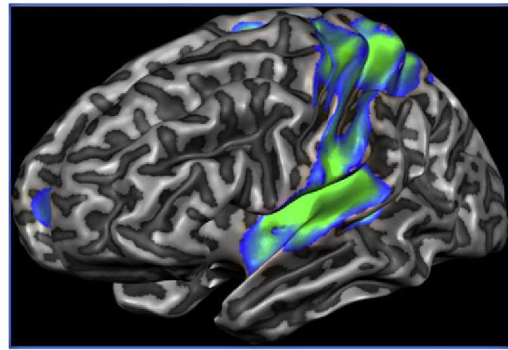
Posterior Insula
