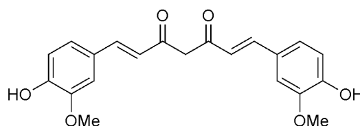
5: Curcumin
