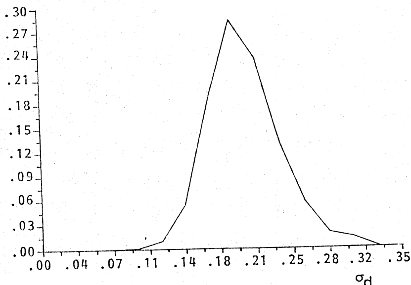
Fig. 5: Marginal posterior density function of \sigma_D .
